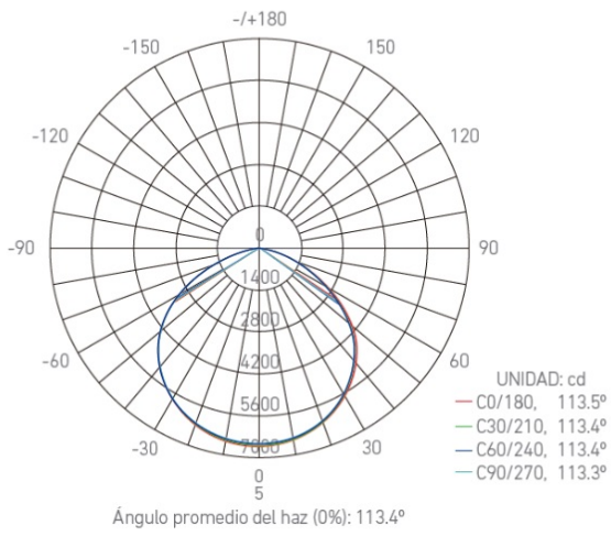
Diagrama Polar
